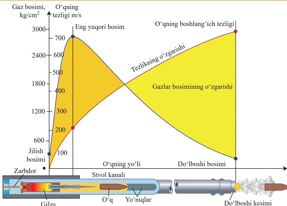
Ichki ballistika. Gazlar bosimining o'zgarishi
