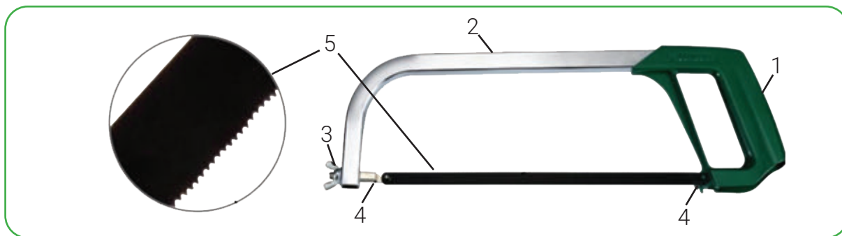
32-rasm. Chilangarlik arrasi tuzilishi: 1 – dasta ; 2 – ramka ; 3 – tortqi vint va quloqli gayka (barashka) ; 4 – shtiftlar ; 5 – polotno (arra) .
