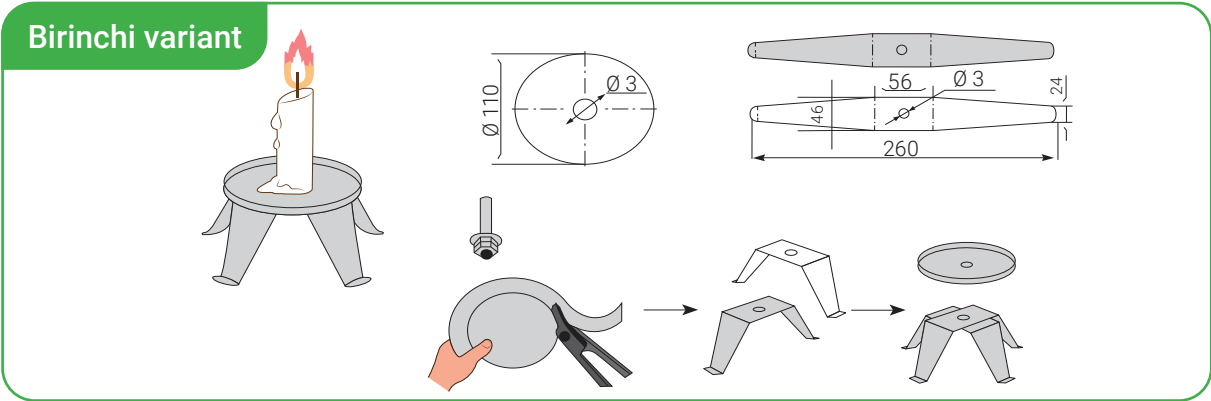
47-rasm. Shamdon yasash texnologiyasi.
