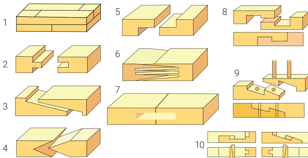
22-rasm. Duradgorlikda qo'llaniladigan ulab uzaytirish usullari: 1 – uchma-uch; 2 – taroqli; 3 – suyri usulda; 4 – ponasimon; 5 – kertmakli; 6 – ponasimon; 7 – qistirma ponali; 8 – ustma-ust qulf usulida; 9 – pog'onali mix cho'pli usulda; 10 – taranglanadigan to'g'ri qulf va qiya usulda.
