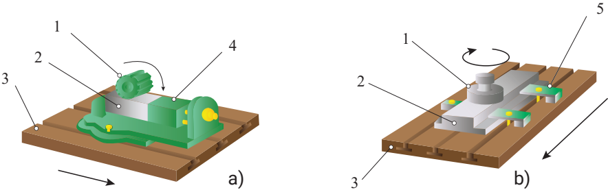
63-rasm. Yuzalarni frezalash: a) zagotovkani tiskida oʻrnatib, silindr freza bilan frezalash; b) zagotovkani stolga oʻrnatib, toresli freza bilan frezalash; bu yerda: 1 – freza; 2 – zagotovka; 3 – stol; 4 – tiski; 5 – qisqich.
